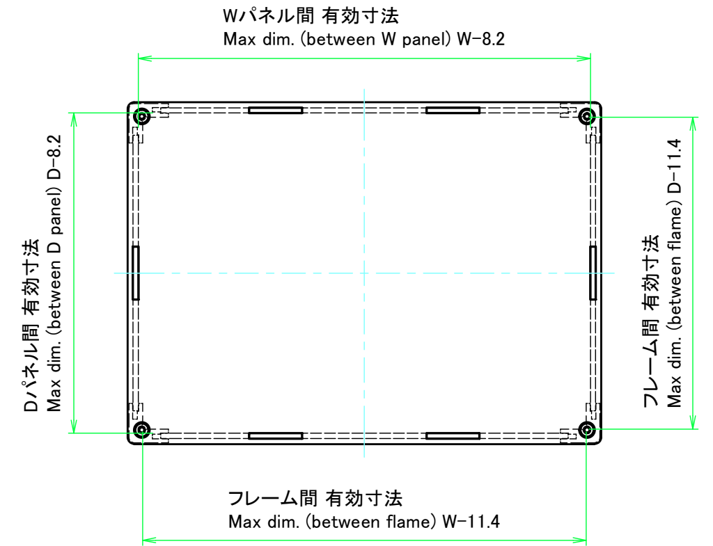
下カバー / Bottom cover
